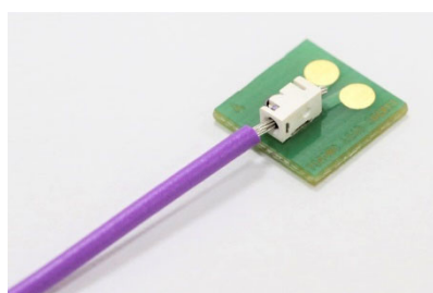
より線対応リードソケット
